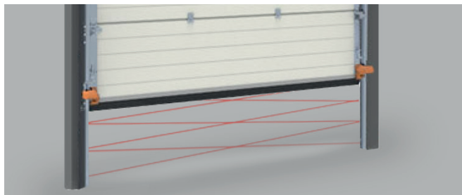
Barrières optiques – conformément à la norme EN 12445 Standard avec automatisation complète
